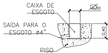
DETALHE DA CAIXA DE ESGOTO (MÁQUINA DE LAVAR SEM ESCALA)
