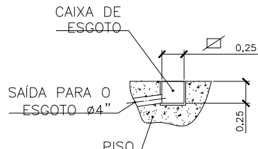
DETALHE DA CAIXA DE ESGOTO (EXTRATOR CENTRÍFUGO SEM ESCALA)
