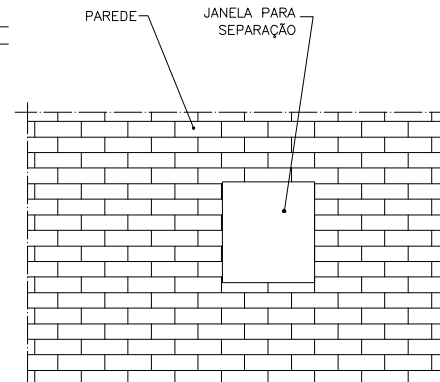
VISTA DE A SEPARAÇÃO DE AMBIENTE (S/ ESCALA)
