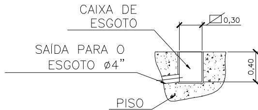
DETALHE DA CAIXA DE ESGOTO (MÁQUINA DE LAVAR SEM ESCALA)
